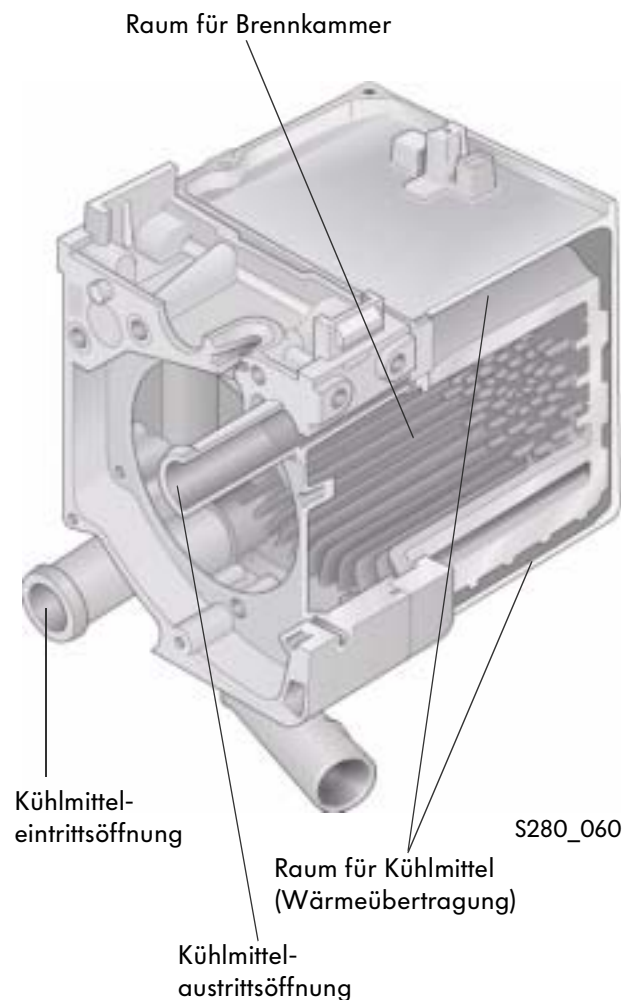
Schnittdarstellung Wassermantel
